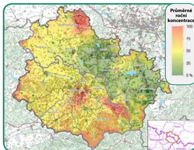
Vliv lokálních topenišť na průměrné roční koncentrace PM_{10} .
