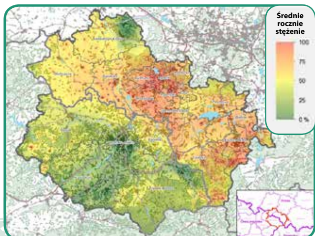
Wpływ przemysłowych źródeł na średnie roczne stężenie PM_{10} .
