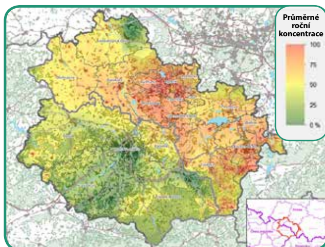
Vliv průmyslových zdrojů na průměrné roční koncentrace PM_{10} .
