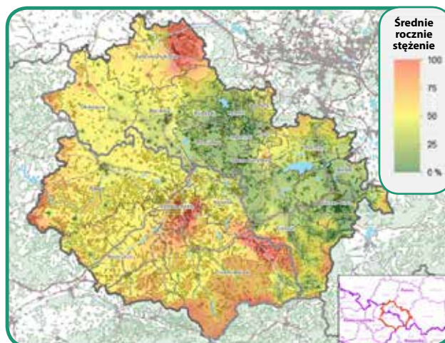
Wpływ ogrzewania domowego na średnie roczne stężenie PM_{10} .
